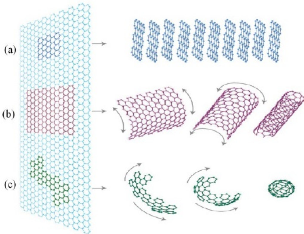
Figura 2.4: Grafeno como uma estrutura base para a formação do: (a) grafite, (b) nanotubos de carbono e (c) fulereno.
