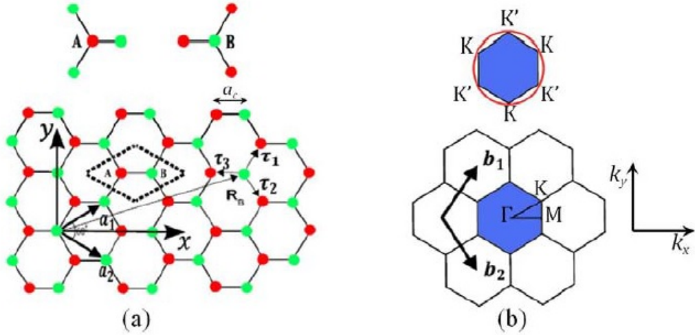
Figura 2.5: Em (a), temos a rede direta do grafeno. O losango representa a célula unitária com os dois sítios inequivalentes: o sítio A em vermelho e o sítio B em verde. \mathbf{a}_1 e \mathbf{a}_2 são os vetores primitivo da rede direta e \tau_1, \tau_2, \tau_3 são os vetores vizinhos mais próximos. Em (b), temos a primeira zona de Brillouin destacada em azul; os vetores primitivos da rede recíproca \mathbf{b}_1, \mathbf{b}_2 e os pontos de simetria \Gamma, M, K e K' .
