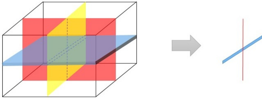
Figura 4.4: Configuração para três campos, resultante da modificação do superpotencial.
