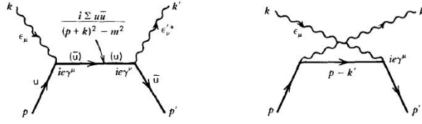
Figura 8 – Diagramas de Feynman para o espalhamento Compton ( e^- \gamma \rightarrow e^- \gamma ). Fonte: Ref. [19].
