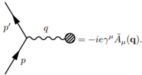
Figura 12 – Espalhamento Coulomb. Fonte: Ref. [23].
